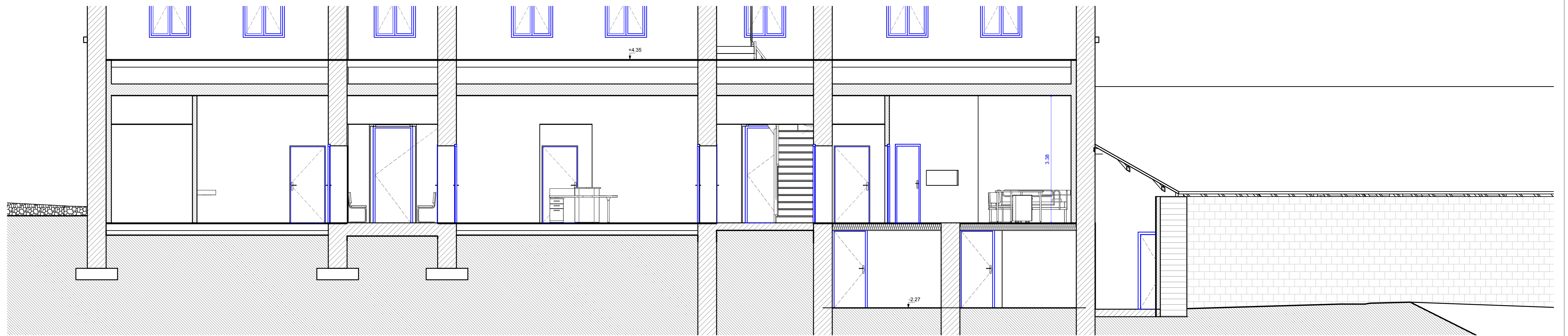
1 Coupe E Echelle : 1 : 50
