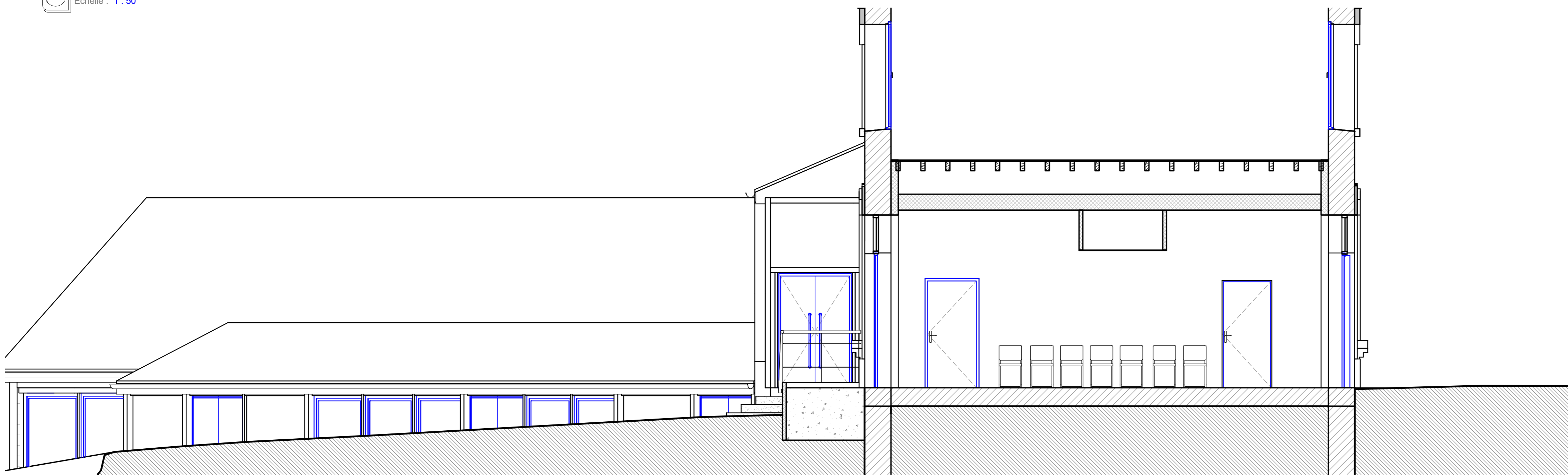
3 Coupe G Echelle : 1 : 50
